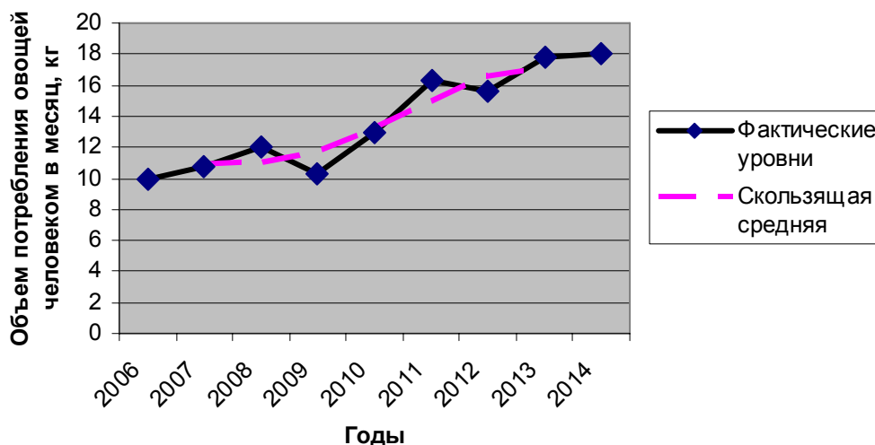
Рис. 6.2. Ряд динамики и линия тренда объема потребления овощей человеком в месяц, кг
