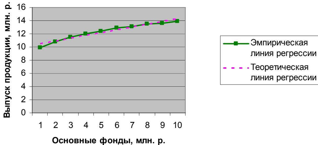
Рис. 8.1. Эмпирическая и теоретическая линия регрессии
