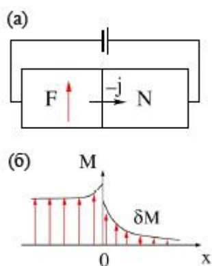
Рис.4.10. (а) Схема прибора для демонстрации концепции электрической спиновой инжекции из ферромагнетика (F) в нормальный металл (N); (б) намагниченность в зависимости от координаты – неравновесная намагниченность \delta M (спиновое накопление) инжектируется в нормальный металл
