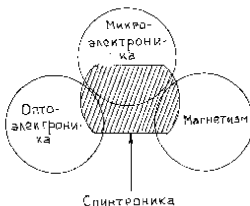
Рис. В.1. Место спинтроники в физике конденсированного состояния
