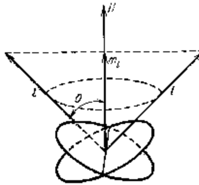
Рис.1.4. Прецессия электронной орбиты ( l ) вокруг магнитного поля ( H )
