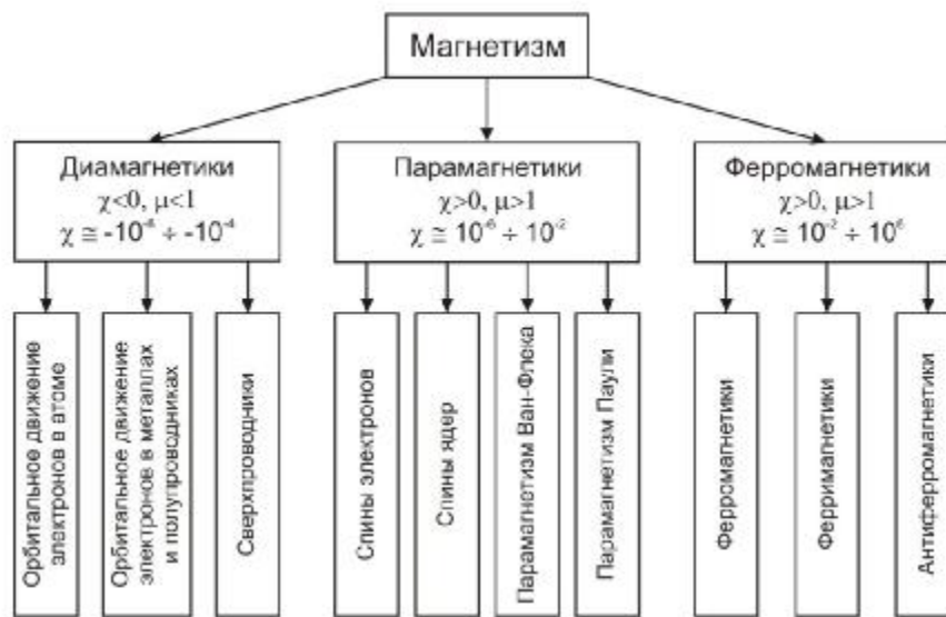
Рис.2.1. Классификация магнетизма
